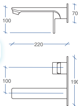
Lavabo empotrado Lux
